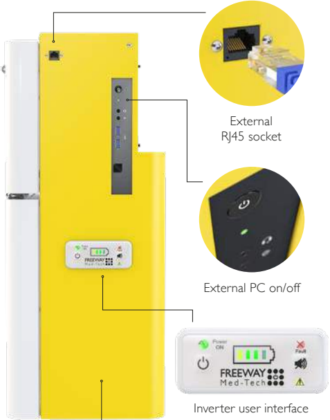
Pod side
